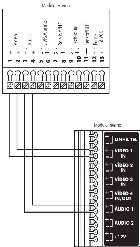
Instalação de áudio e vídeo
