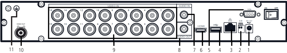
Painel posterior MHDX 5216
