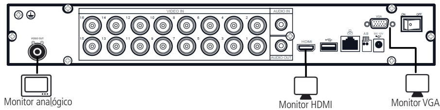
Saídas de vídeo
