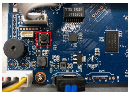
Botão de reset
