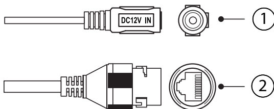
Cabo multifunções VIP 3230 W e VIP 3430 W
