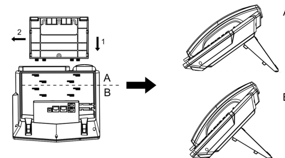
Montagem do pé na base do terminal IP V5501
