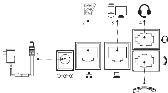
Visão posterior das conexões do terminal IP V5501
