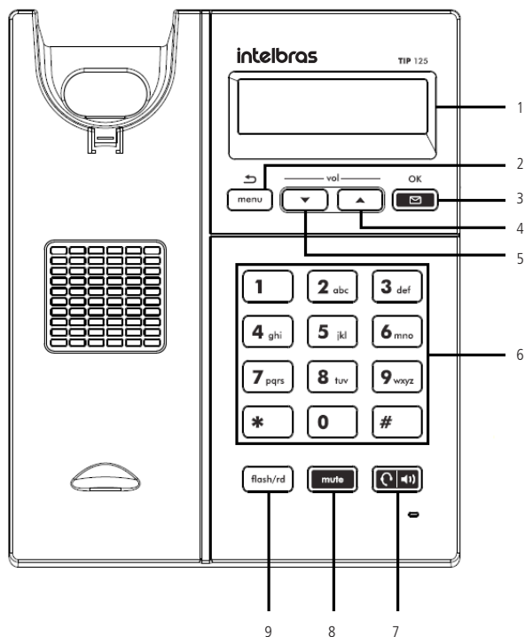
Visão frontal
