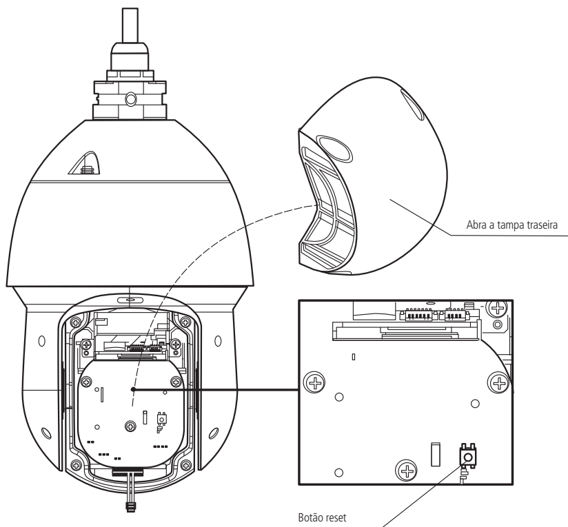
Botão de reset VIP 3212 SD IR
