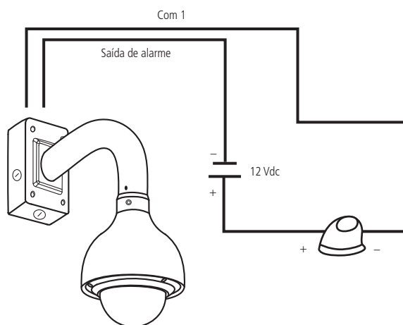
Conexão dos dispositivos de alarme
