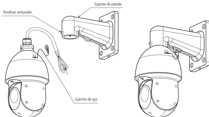
Instalação do suporte
