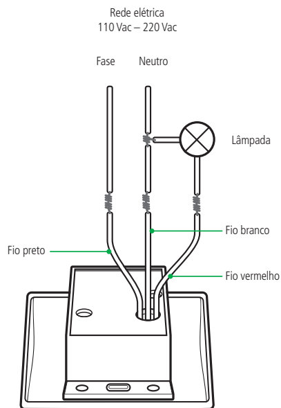
Conexões elétricas
