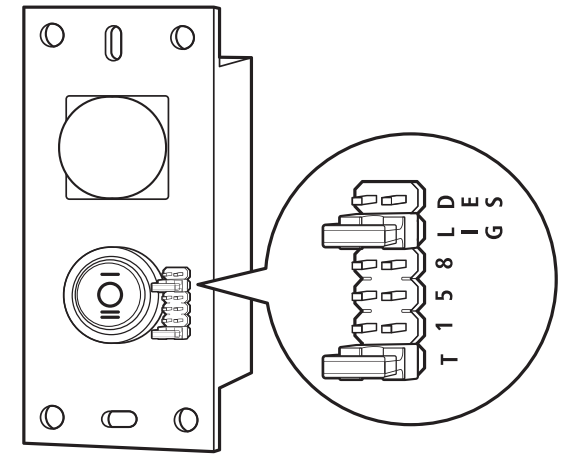
Jumpers de configuração
