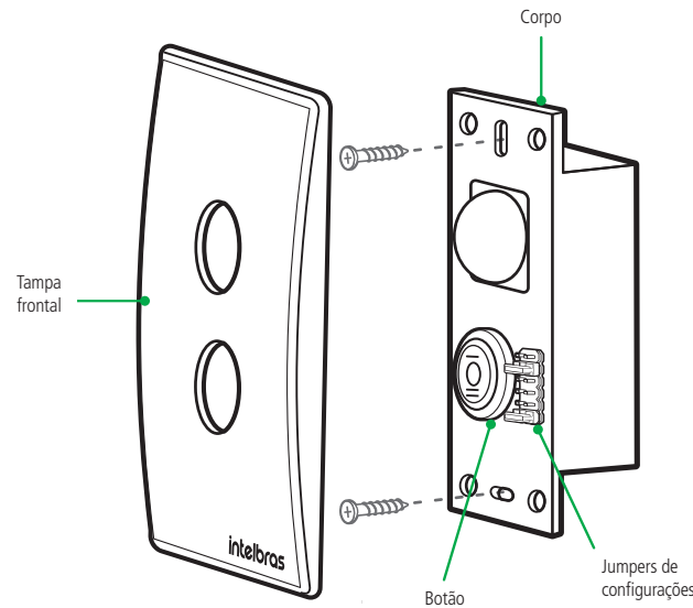
Tampa frontal e corpo do sensor
