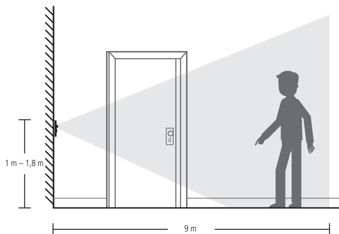
Altura de instalação e distância máxima de detecção
