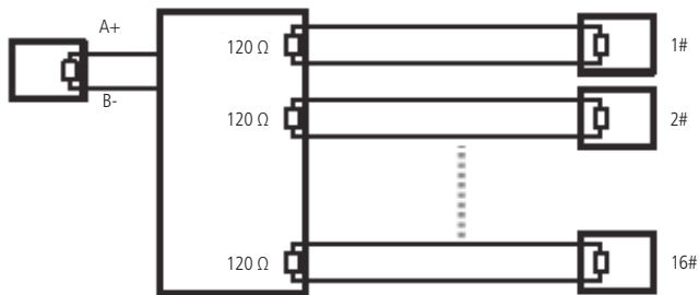
Distribuidor RS485
