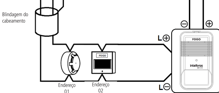
Conexão da saída 24 V
