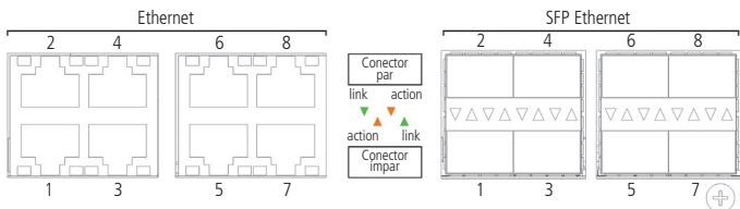
Vista frontal LEDs das portas GE
