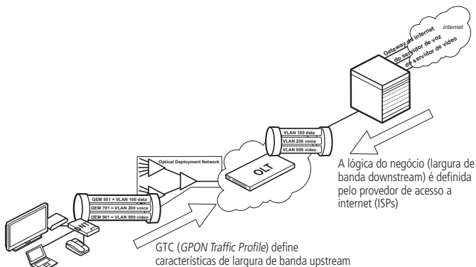
Solução GPON
