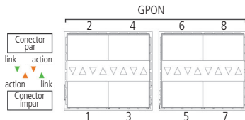
Vista frontal – LEDs das portas 10 GE
