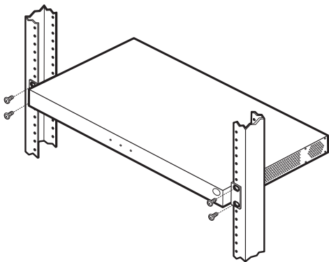
Instalando a OLT 8820 I em rack 19"
