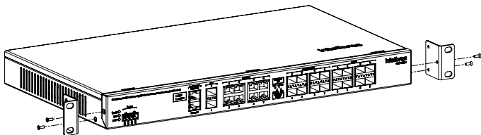
Instalando os suportes de fixação
